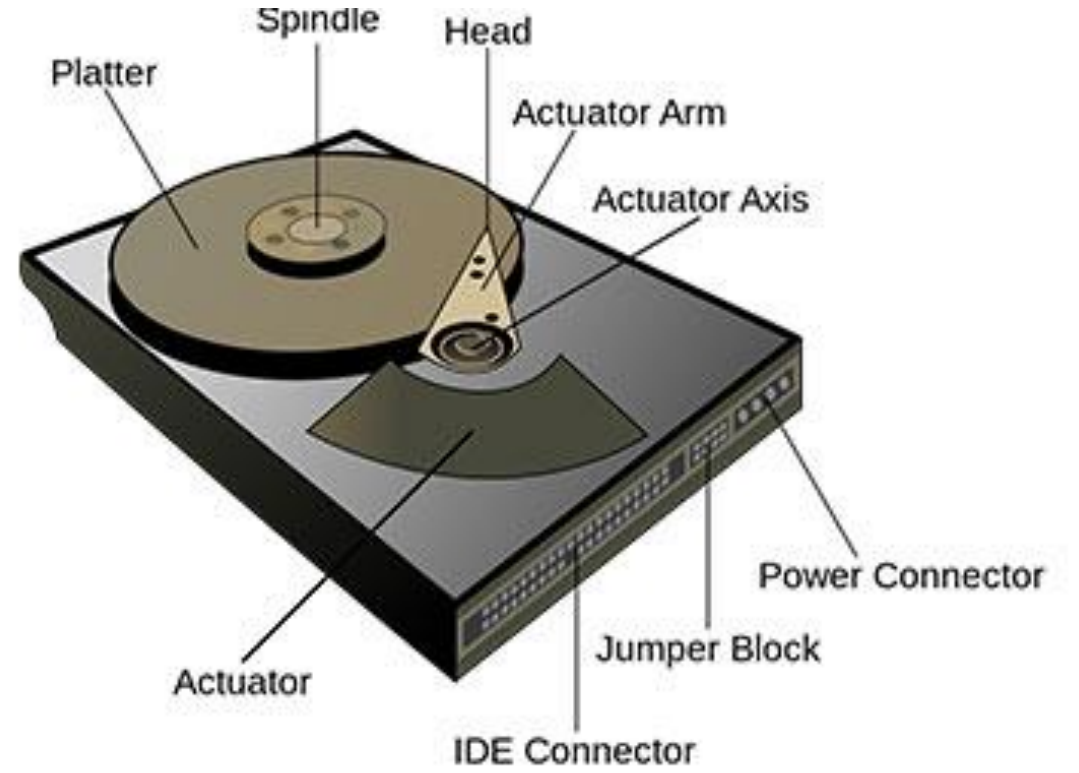
HDD
