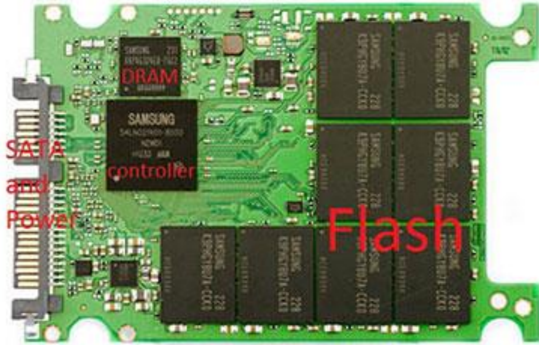
SSD
